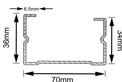
DF-GI-Stud - 70mm Premium
