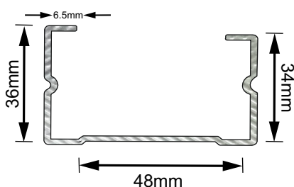
DF-GI-Stud - 48mm Premium
